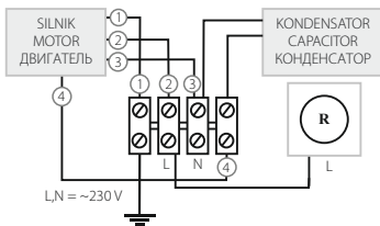
SCHEMAT PODŁĄCZENIA CONNECTION SCHEME / СХЕМА ПОДКЛЮЧЕНИЯ REGULATOR OBROTÓW / SPEED CONTROLLER / РЕГУЛЯТОР ОБОРОТОВ WK
